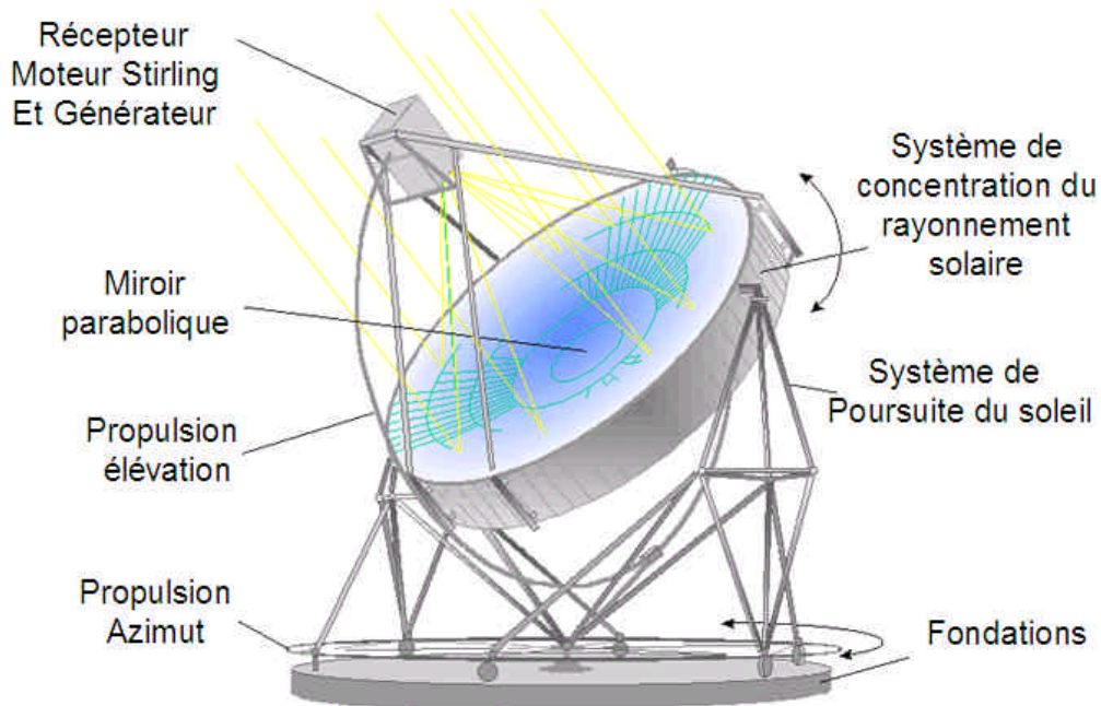
Figure 3 : Système Dish/Stirling
